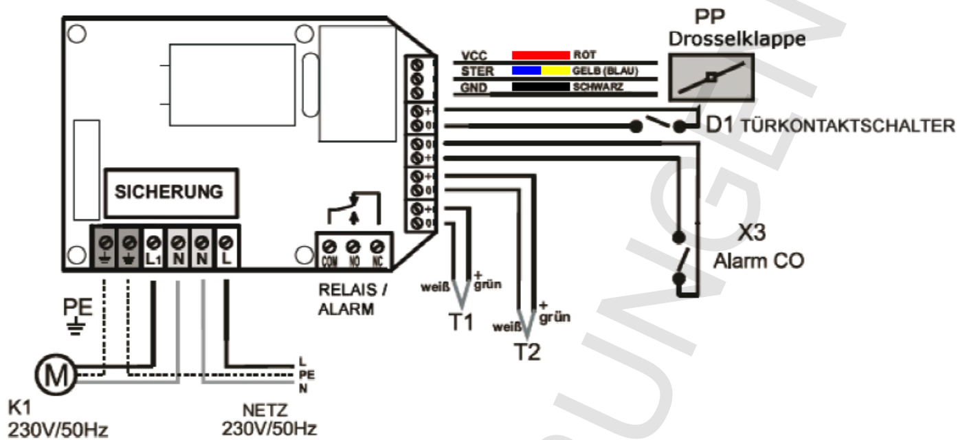
Abb.2 - Elektroinstallationschema
